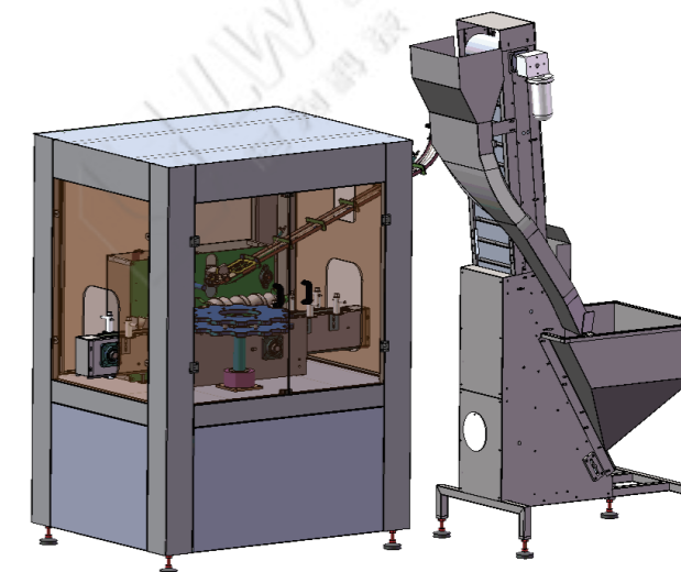
压盖机 LW-CPC350 LID PRESS CAPPING MACHINE LW-CPC350
